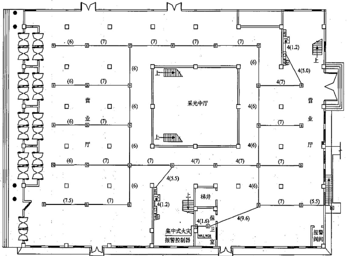
图 3-3A 一层消防报警及联动平面图
