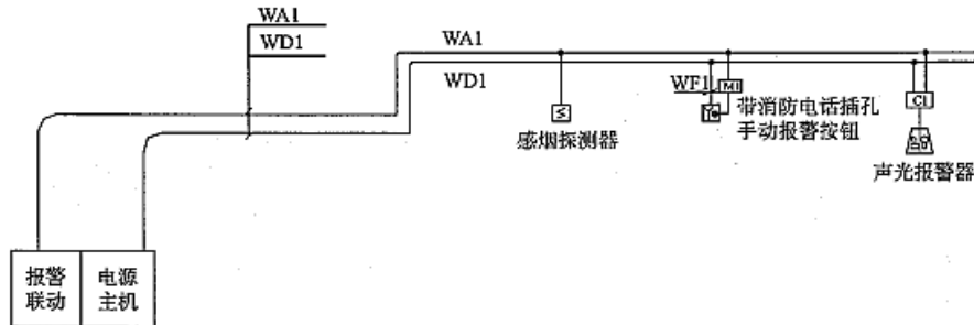
图 3-3B 火灾自动报警及广播系统图
